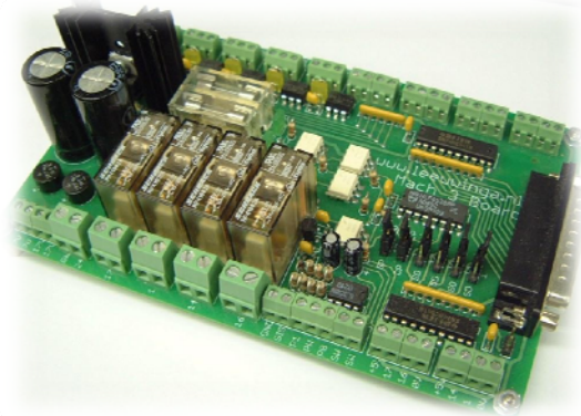
Mach3 interface kaart CD9430
