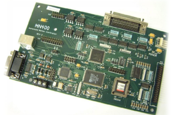
MN400 interfacekaart in microtechniek uitgevoerd
